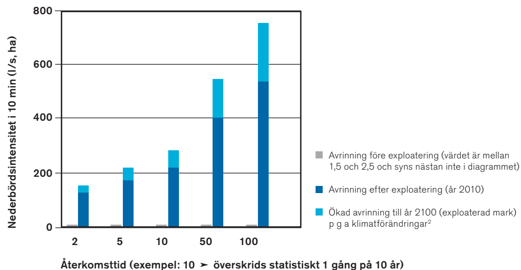
AVRINNING FÖRE & EFTER EXPLOATERING (100% HÅRDCJORT)
